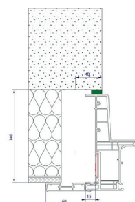
Demi-linteau
